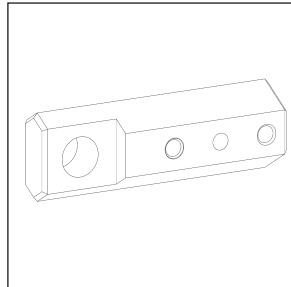
Position 31 | 1×
