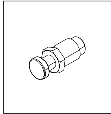
Position 6 Index Plunger M30x1.5 (1x)
